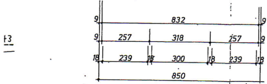
ERDGESCHOSS
