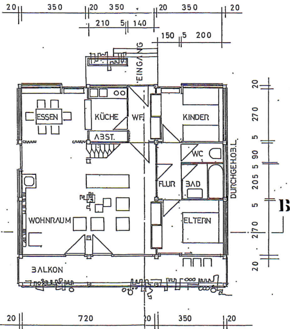
ERDGESCHOSS
