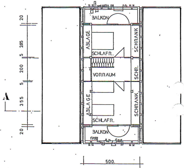
OBERGESCHOSS
