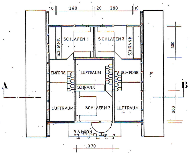
OBERGECHOSS
